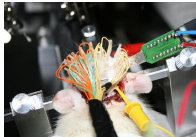
ラット用EEG装置
