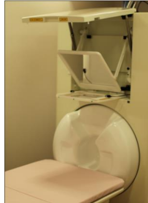
200チャンネル MEG装置
